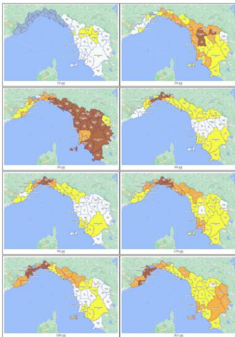
Distribuzione areale indice SPI (2022-06-07)
